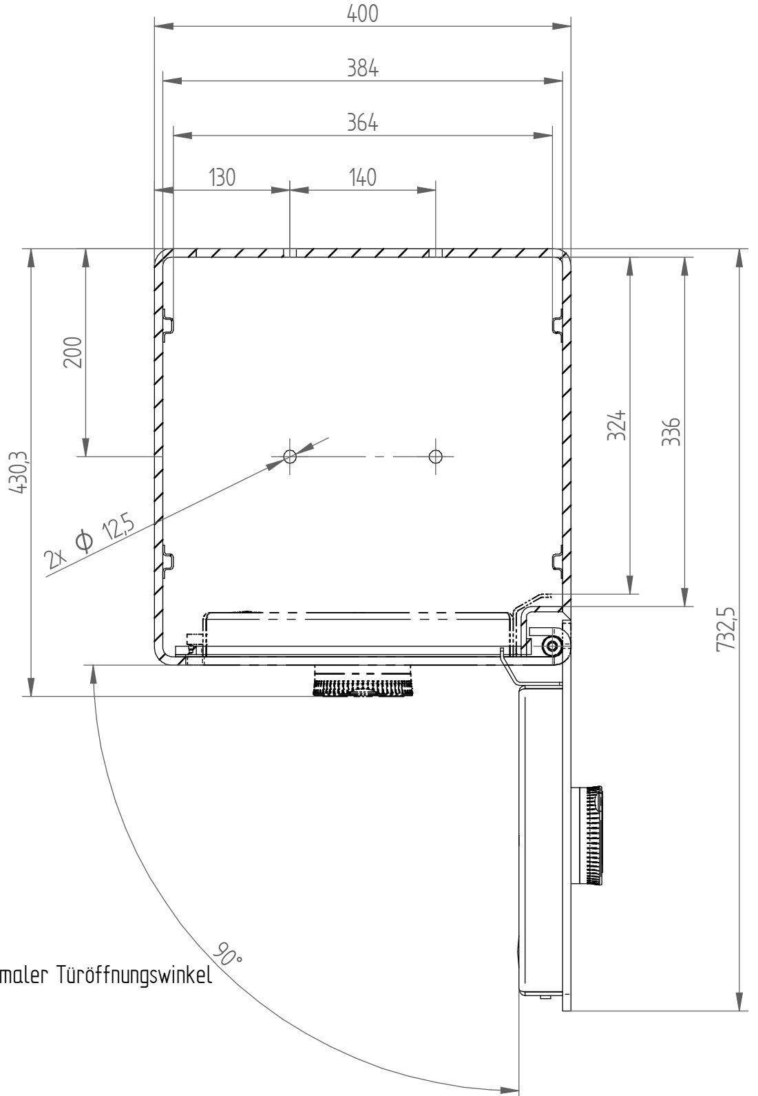
Schnitt B-B
