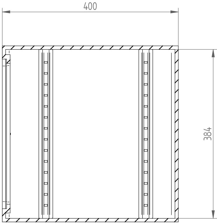
Schnitt A-A
