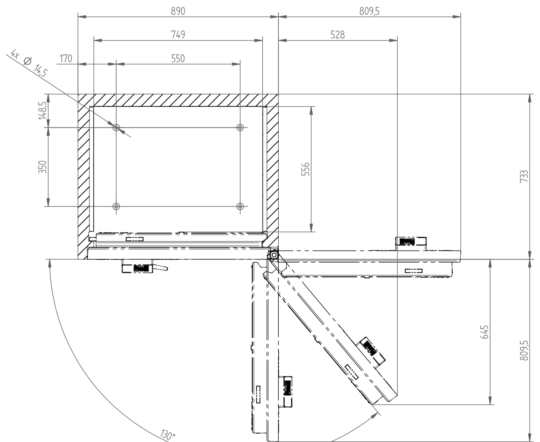
Schnitt A-A
