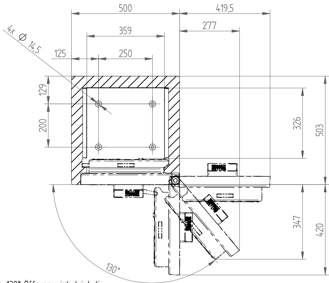
Schnitt A-A
