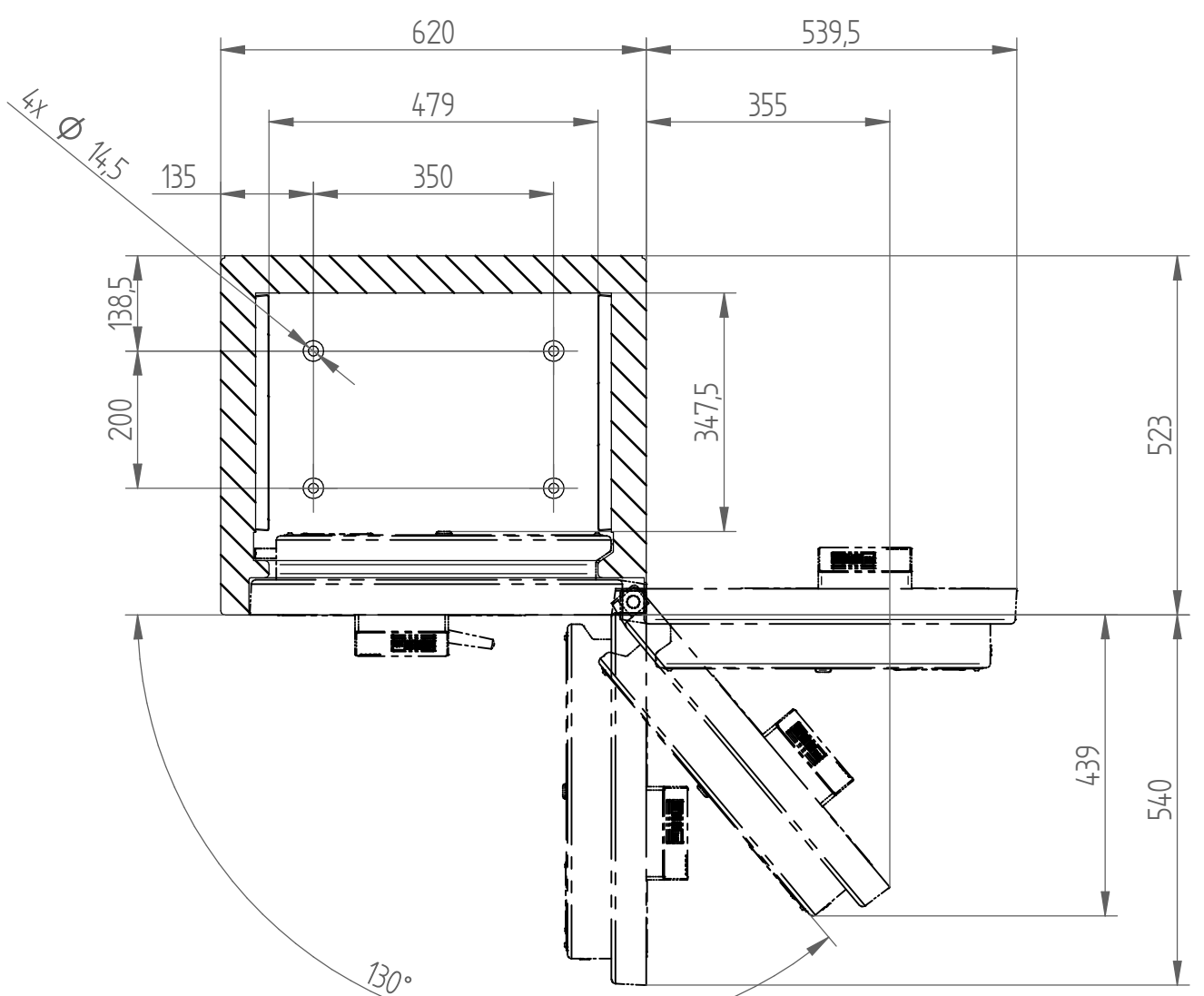
Schnitt A-A
