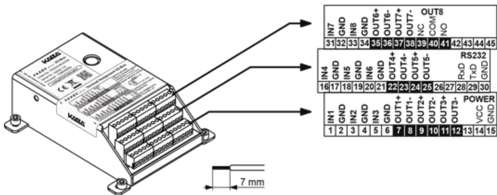
Klemmenbelegung I/O-Box
