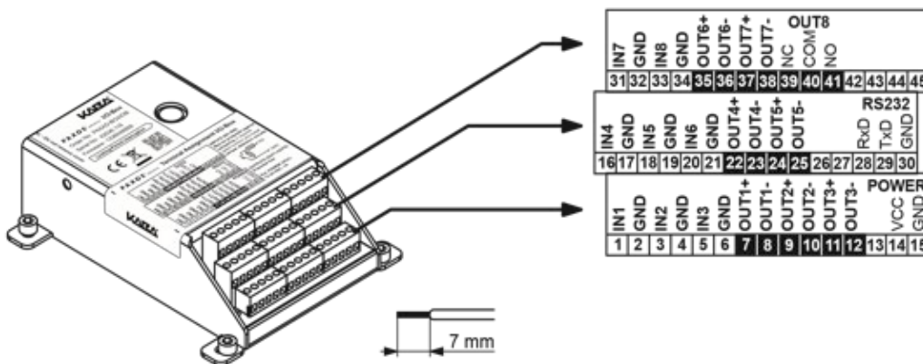
Klemmenbelegung I/O-Box
