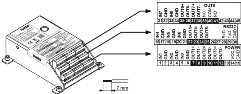
Klemmenbelegung I/O-Box
